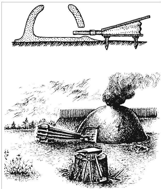
Металлургический горн. Реконструкция Ю. А. Семькина
