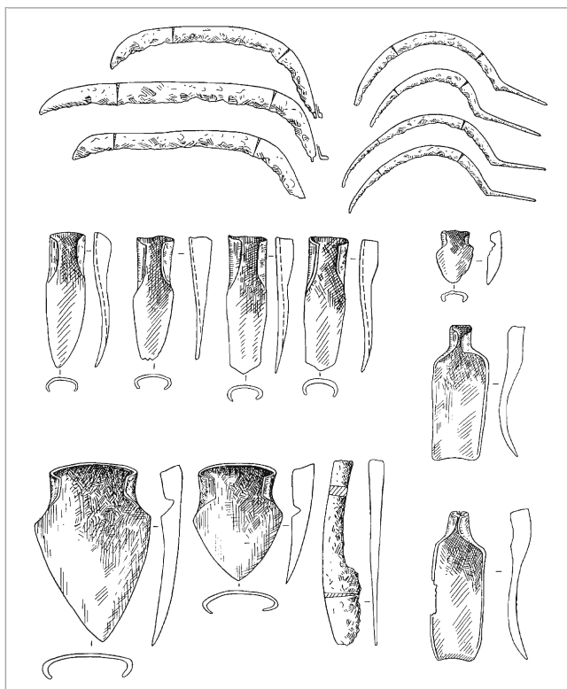
Земледельческие орудия труда: косы, серпы и де- тали плуга
